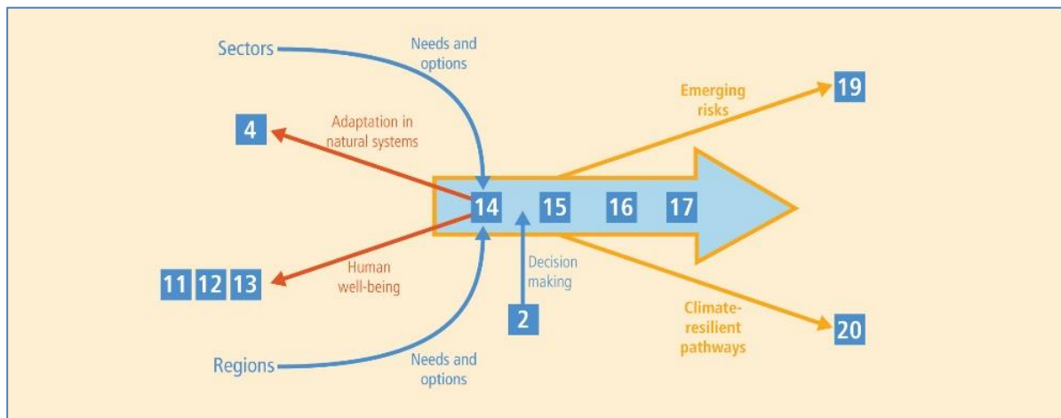
Figure 1 (issue de la figure 14-1 de l'AR5). Les quatre chapitres sur l'adaptation (14 à 17) sont étroitement liés à plusieurs autres chapitres. Le chapitre 14 (Besoins et options d'adaptation) aborde et recoupe de nombreuses questions relatives au bien-être humain, y compris la santé, la sécurité et la pauvreté ; le traitement de l'adaptation des écosystèmes naturels est traité principalement au chapitre 4 et n'est pas repris au chapitre 14. De même, les besoins et options synthétisés au chapitre 14 sont largement tirés des chapitres sectoriels (3 à 10) et régionaux (21 à 30). Le chapitre 2 fournit des informations sur les approches décisionnelles pertinentes au chapitre 15 (Planification et mise en œuvre de l'adaptation). Tous les chapitres sur l'adaptation alimentent la synthèse des chapitres 19 (Risques émergents et principales vulnérabilités) et 20 (Voies résilientes au changement climatique : adaptation, atténuation et développement durable) (p. 838 – AR5 – traduction de l'auteur).
